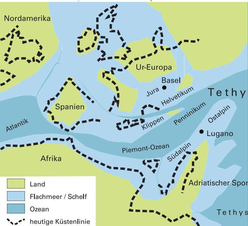
1. vor 140 Millionen Jahren: Ablagerung der Sedimente im Ur-Mittelmeer Tethys
